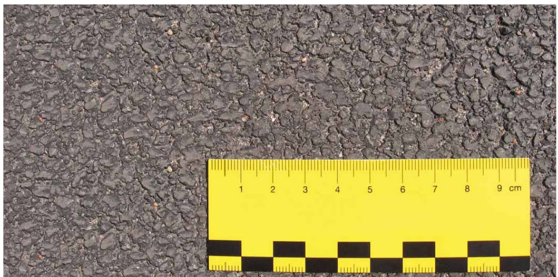
Durch eine verringerte Grobtextur der Asphaltoberfläche lassen sich die Geräuschemissionen im Straßenverkehr vermindern. Der speziell für die Stadt Düsseldorf entwickelte Asphalt besitzt daher ein Größtkorn von nur 5 mm.
